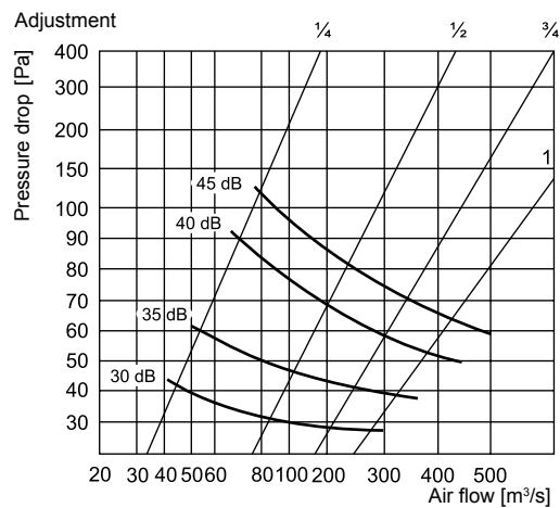
P-DVS 200
